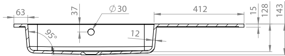
PRZEKRÓJ N-N
