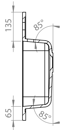
PRZEKRÓJ M-M
